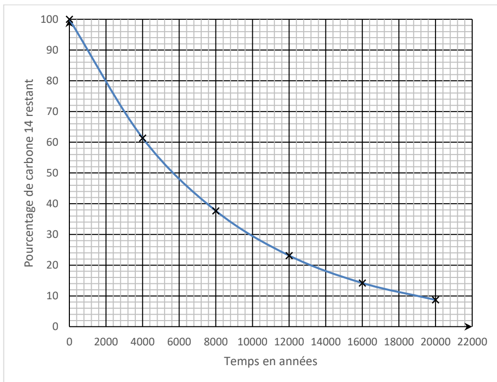
Figure1 : courbe de décroissance radioactive du carbone 14
