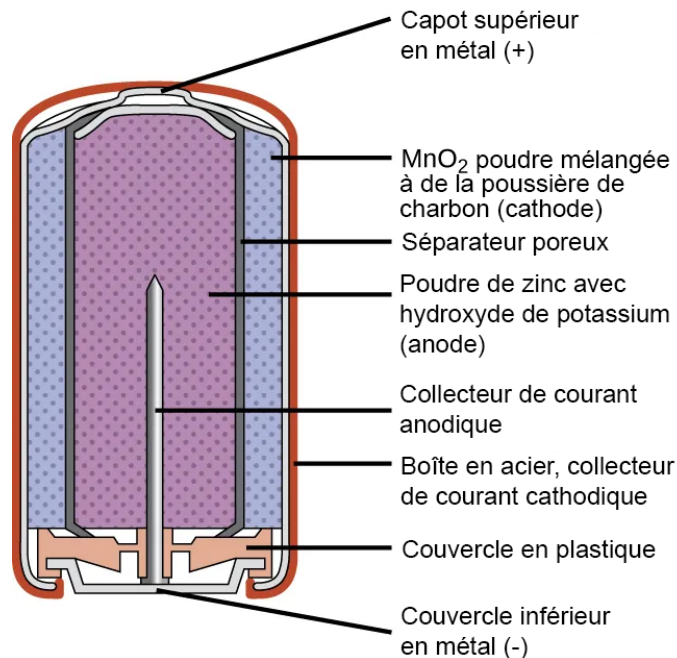
Figure 2 : Schéma d'une pile alcaline (source : Wikipédia)
