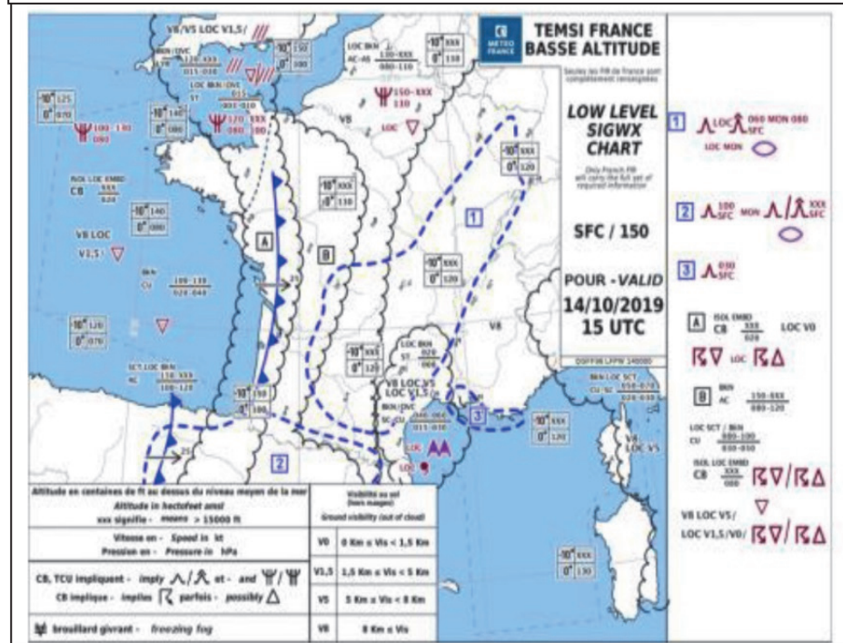
Carte TEMSI
